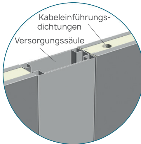
Paneelverbindung mit Versorgungssäule
