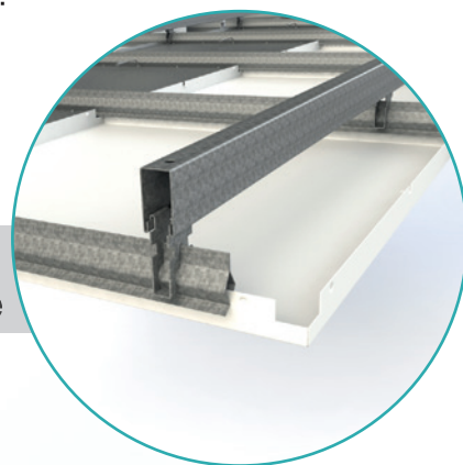
Detailansicht der Hängepaneele
